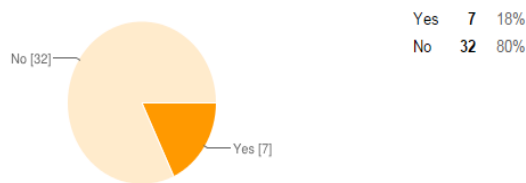
Fig. 13 (Using AOP)
